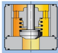
锥阀
